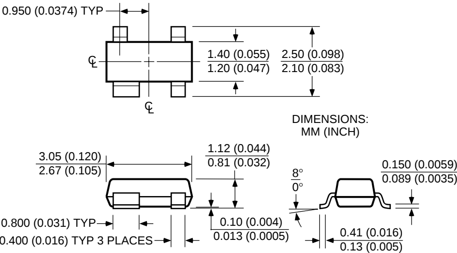
SOT-143 (M4)
